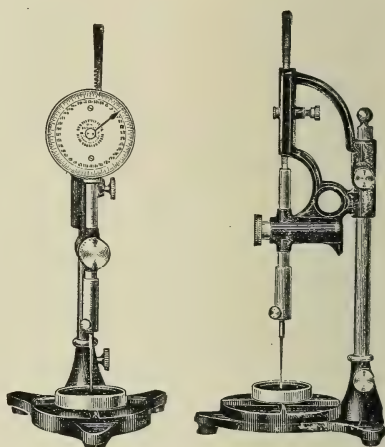
FIG. 164.—Miniature Penetrometer.
